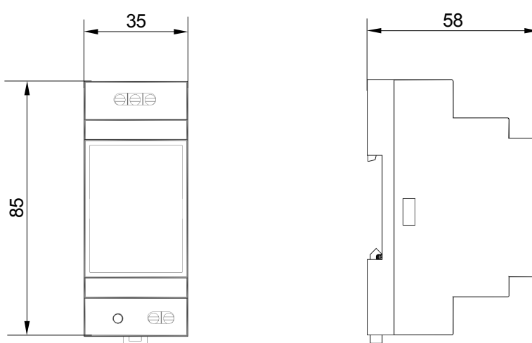
фиг. 2 – габаритни размери
